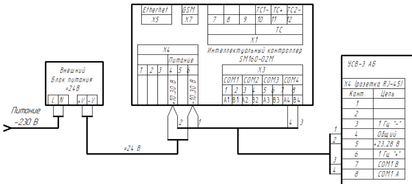
Рисунок Д.2 – Подключение УСВ-3 С АБ к контроллеру SM160-02M
