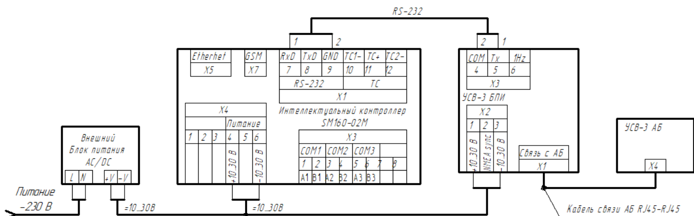
Рисунок Д.1 – Подключение УСВ-3 с АБ и БПИ к контроллеру SM160-02M
