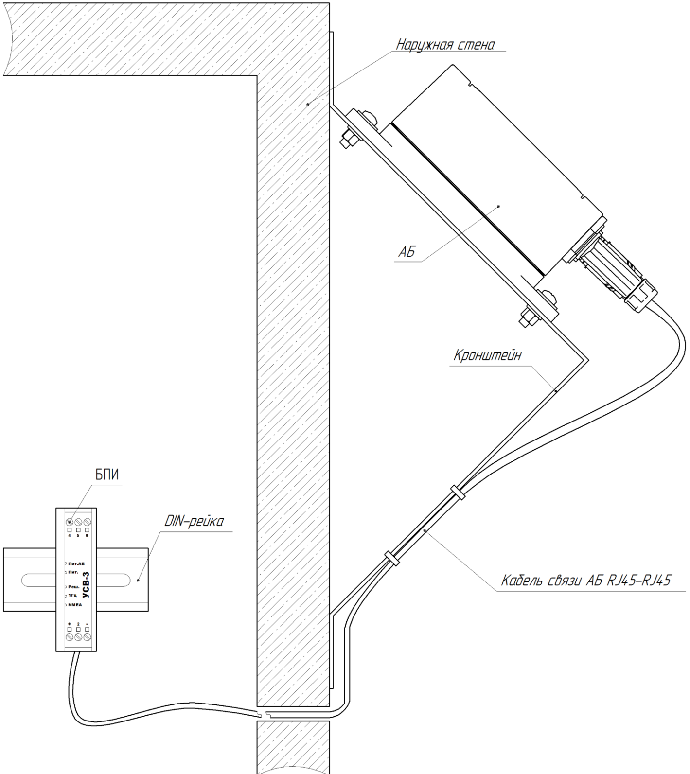
Рисунок Е.1 - Пример монтажа УСВ-3 с АБ и БПИ
