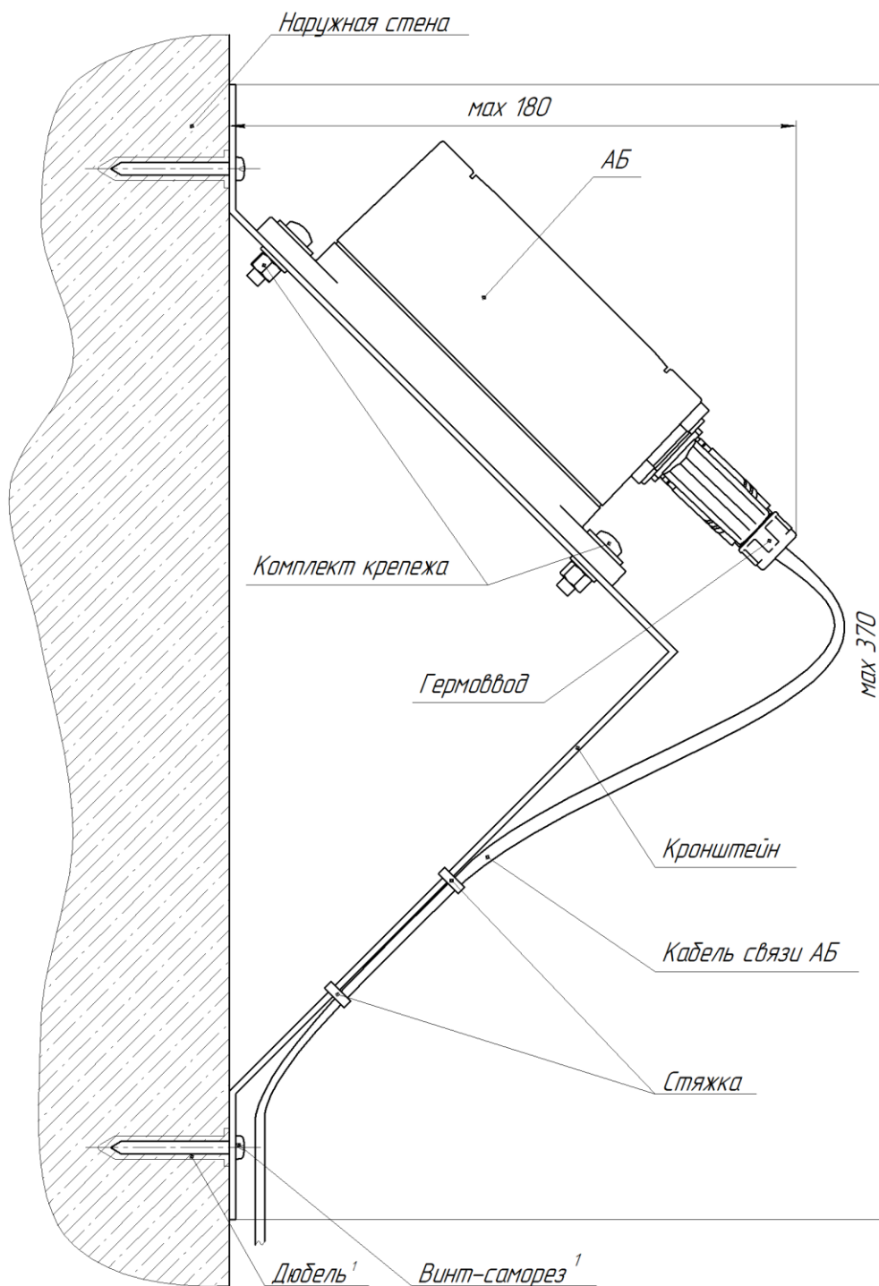
Рисунок Б.1 – Внешний вид АБ с кронштейном
