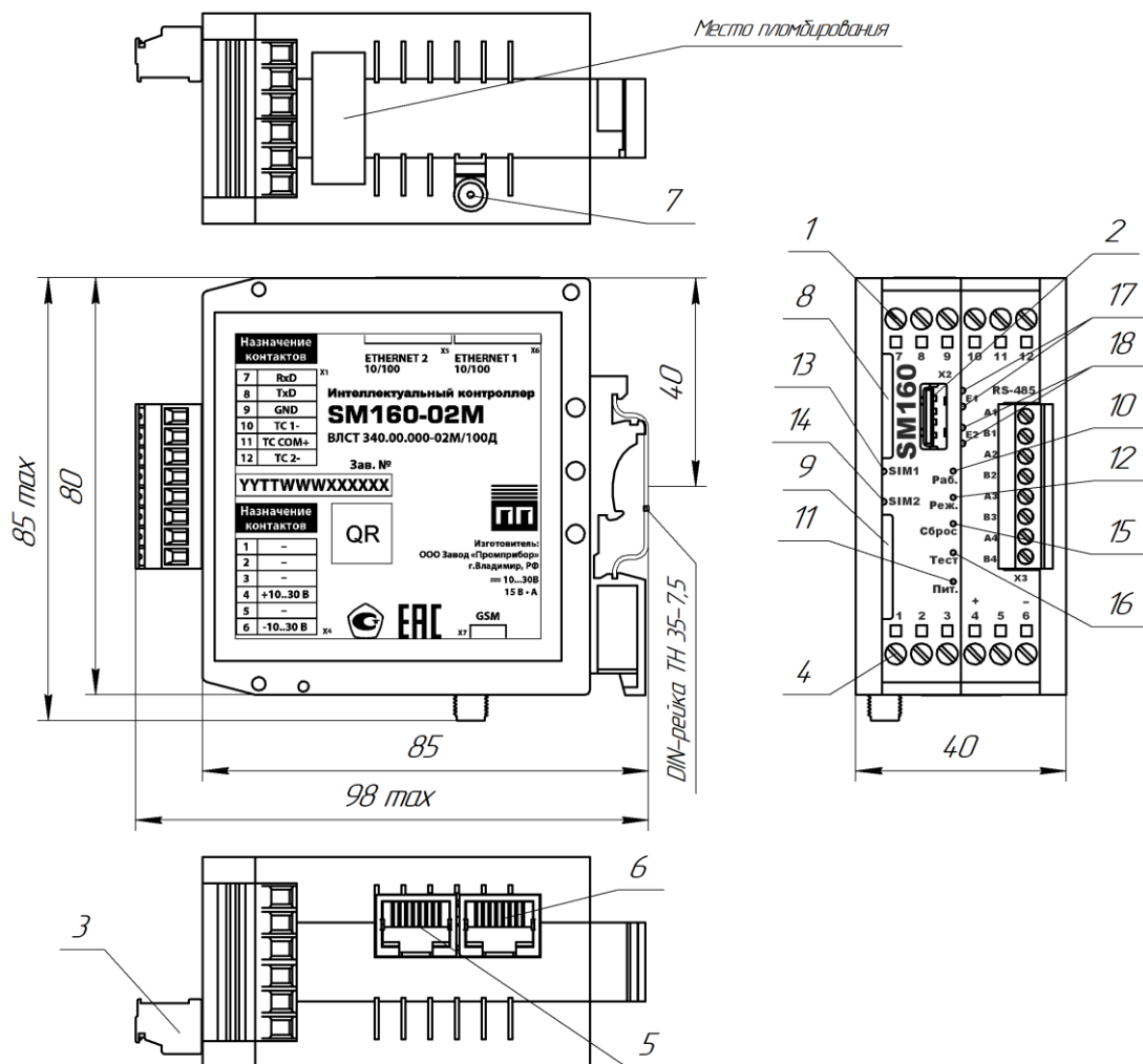
Рисунок А.1 – Общий вид контроллера без СКЗИ Таблица А.1 - Органы коммутации и индикации контроллера
