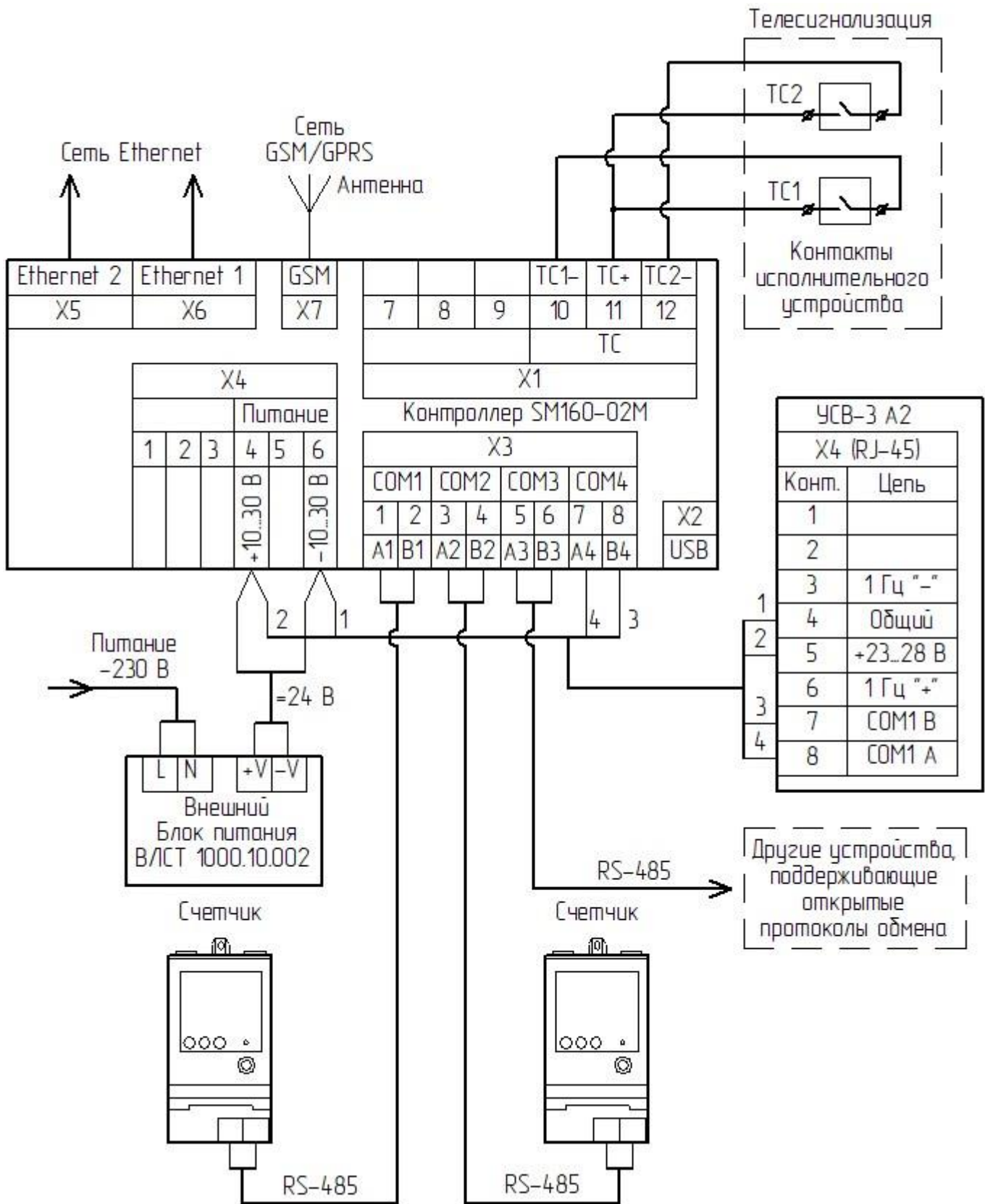
Рисунок Б.2 – Подключение антенного блока УСВ-3 к контроллеру
