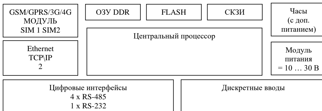
Рисунок 1.1 – Общая структурная схема контроллера
