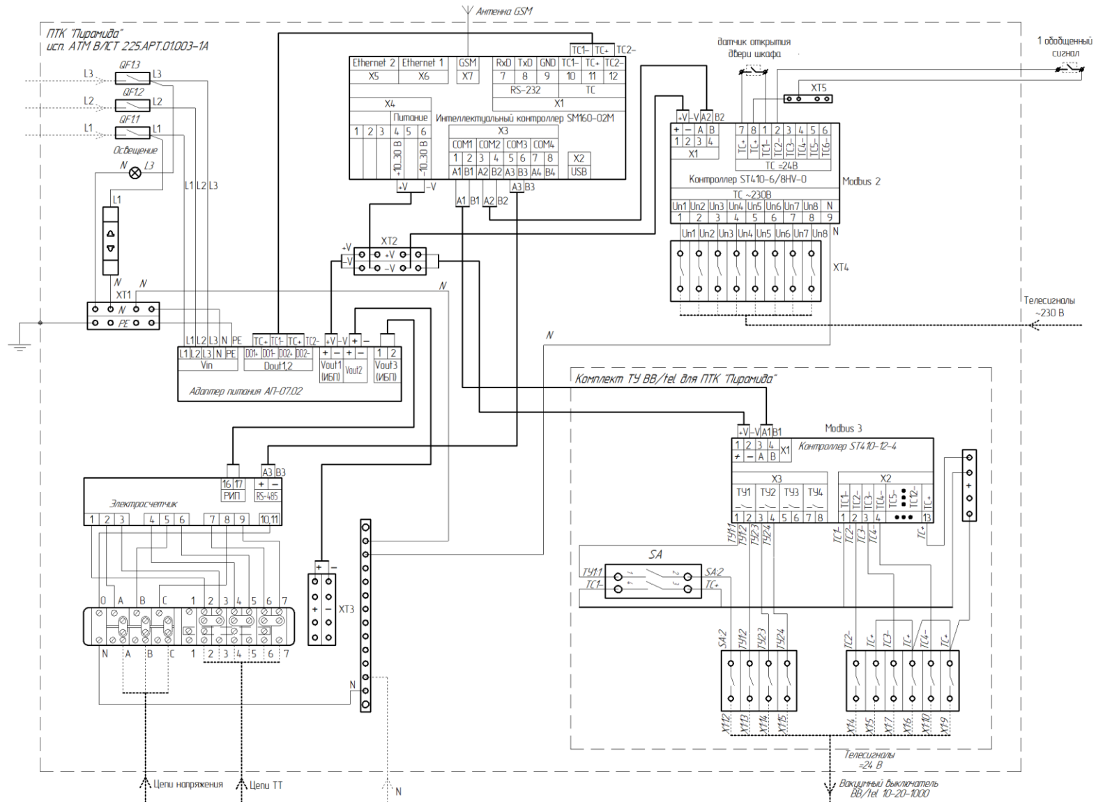
Рисунок Г.1 – ПТК «Пирамида» исп. АТМ ВЛСТ 225.АРТ.01.003-1А
