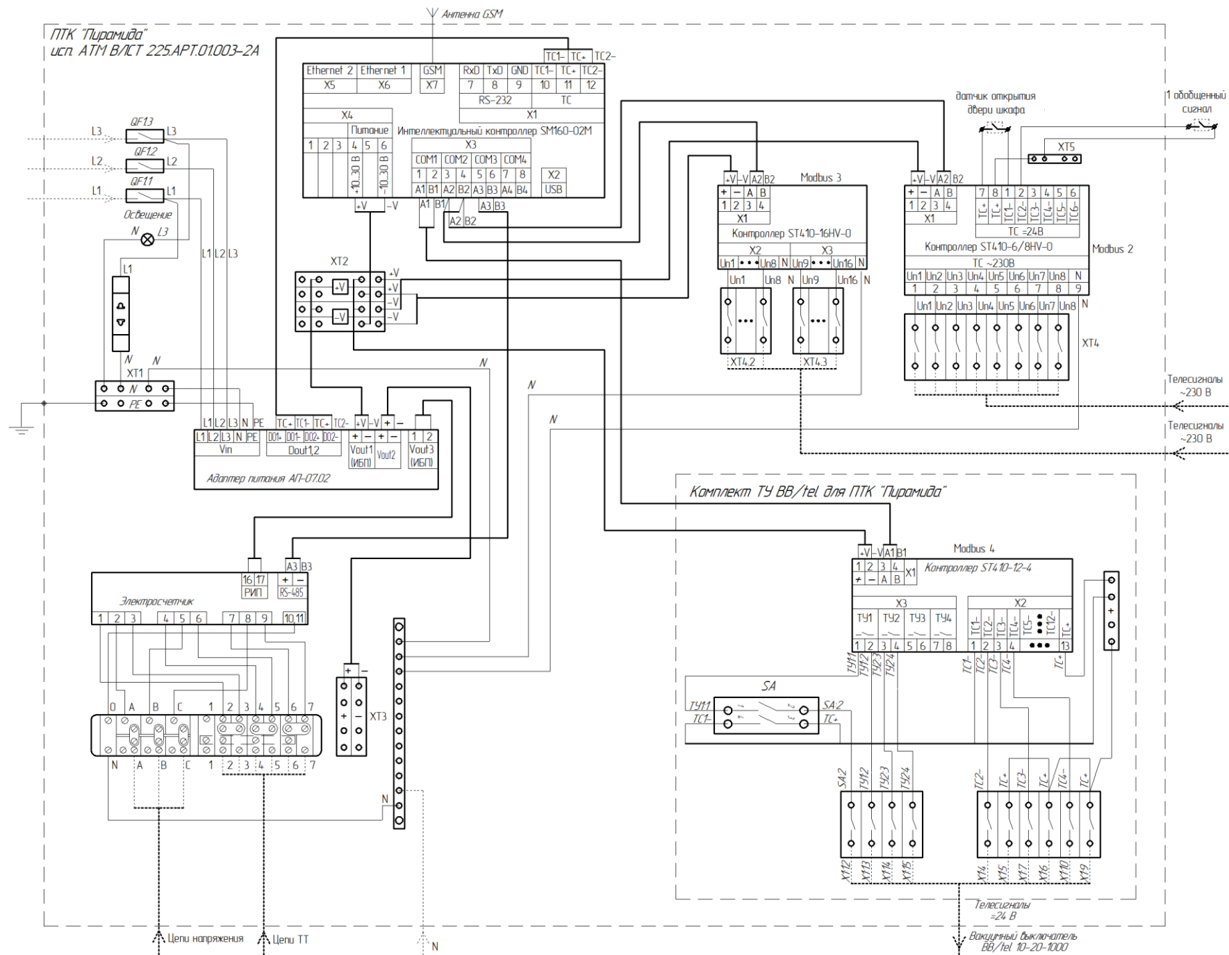
Рисунок Г.2 - ПТК «Пирамида» исп. АТМ ВЛСТ 225.АРТ.01.003-2А
