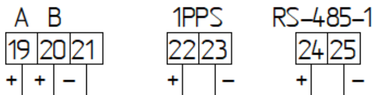
Рисунок А.4 – Подключение сигнальных цепей счетчика непосредственного включения в исполнении W (назначение групп контактов слева направо: активная/реактивная энергия; выход 1PPS; интерфейс RS-485 линия A «+» и линия B «-»)
