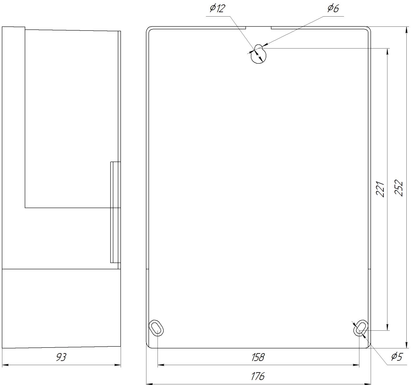
Рисунок Б.1 - Размеры счетчика в исполнении W
