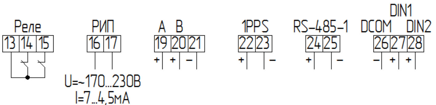
Рисунок А.3 – Подключение сигнальных цепей счетчика трансформаторного включения в исполнении W (назначение групп контактов слева направо: два дискретных выхода; резервный источник питания; активная/реактивная энергия; выход 1PPS; интерфейс RS-485 линия A «+» и линия B «-»; два дискретных входа)
