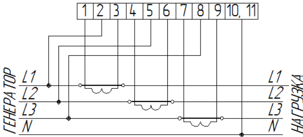
Рисунок А.1 - Схема подключения счетчика непосредственного включения
