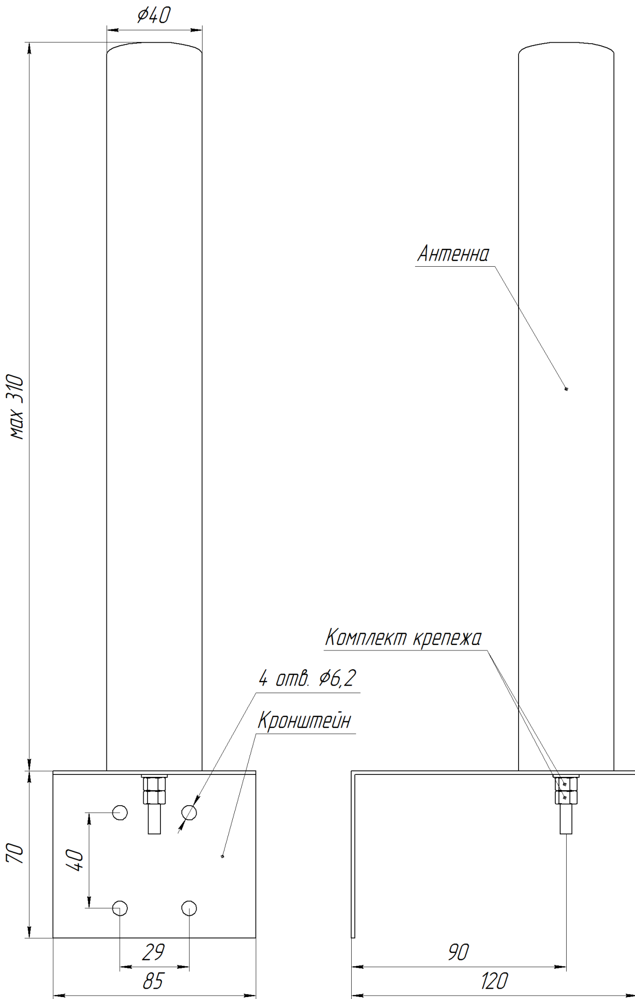
Рисунок 1 – Внешний вид антенны
