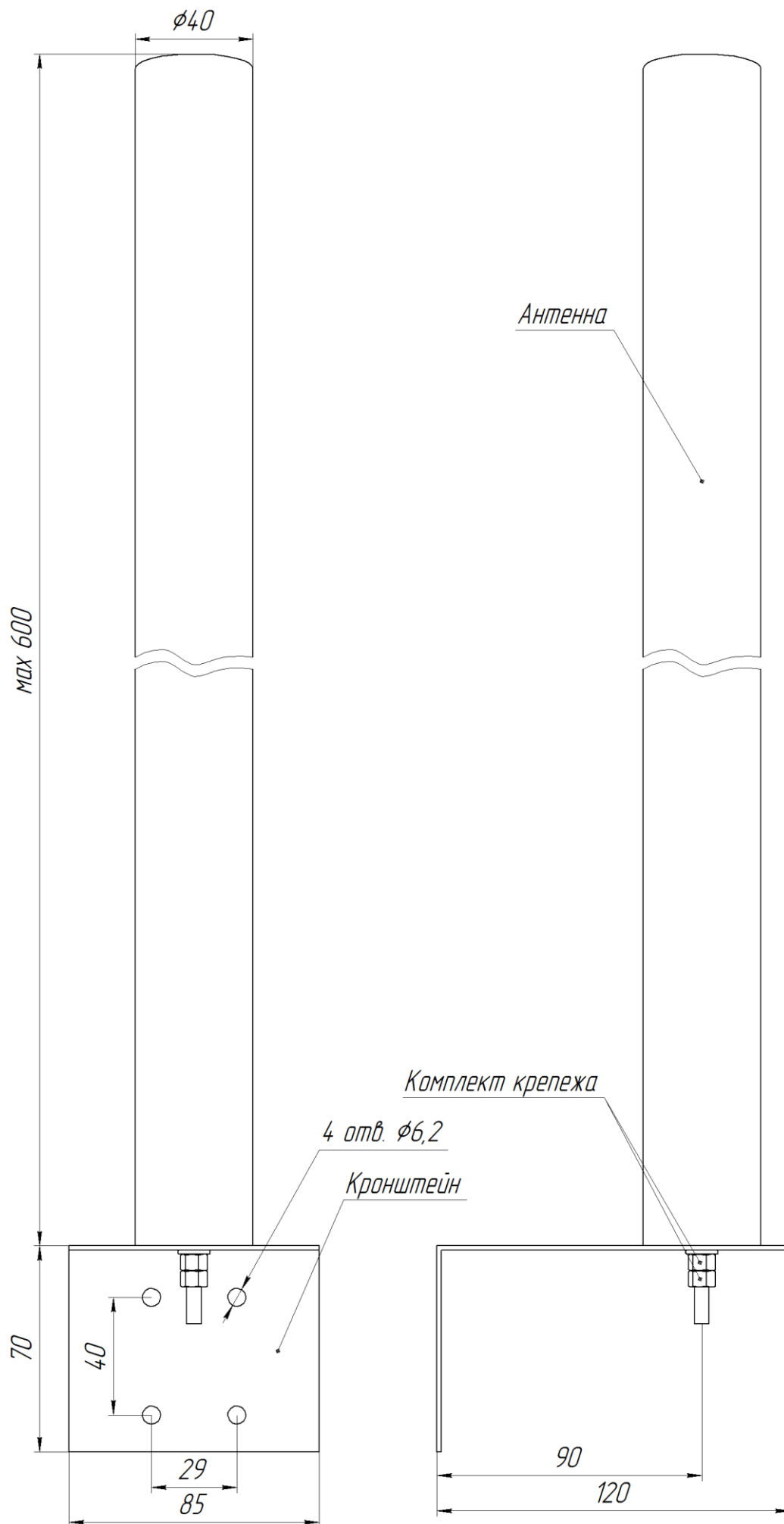
Рисунок 1 – Внешний вид антенны
