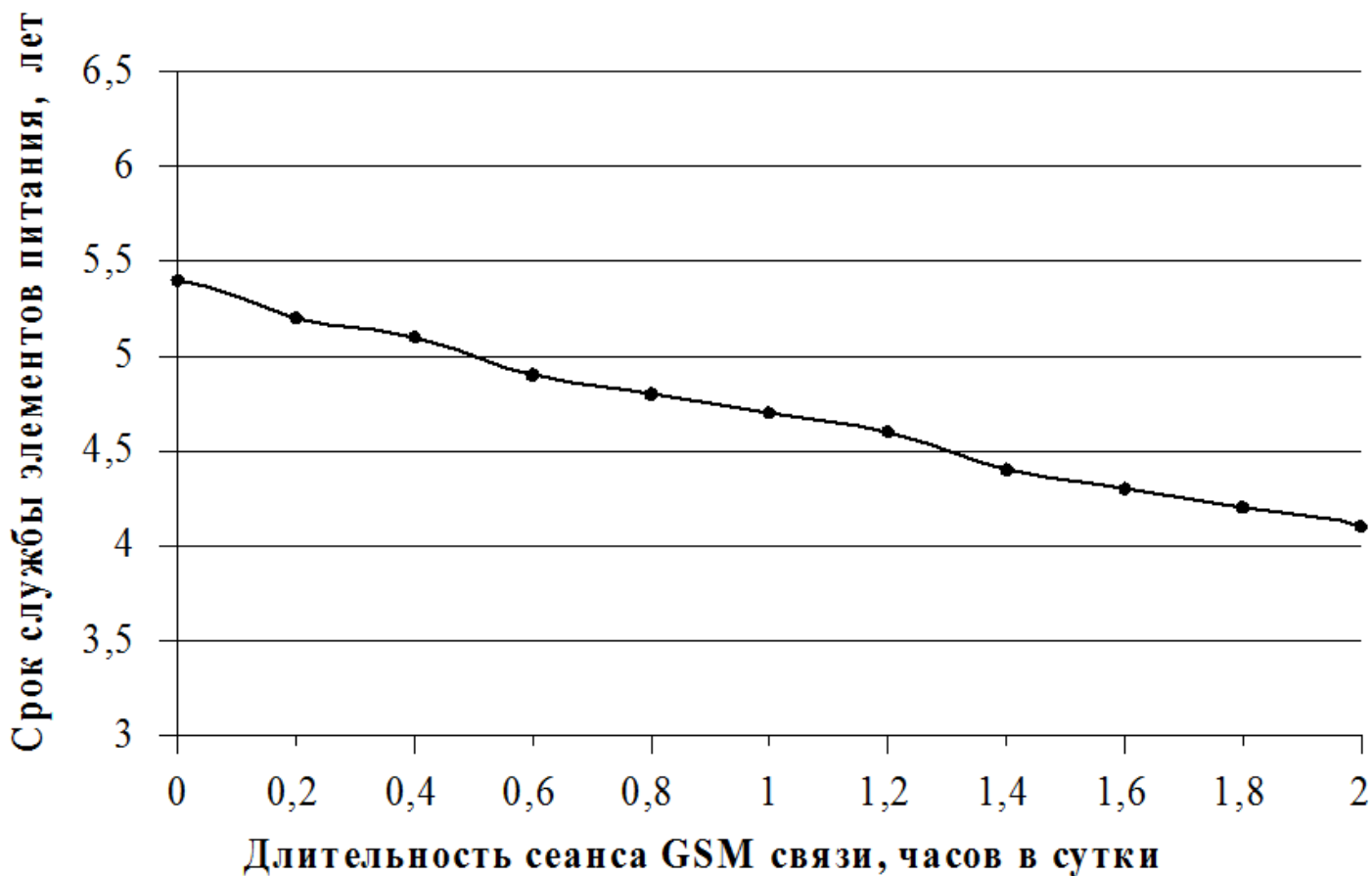
Рисунок 3.1 – Срок службы батарей питания
