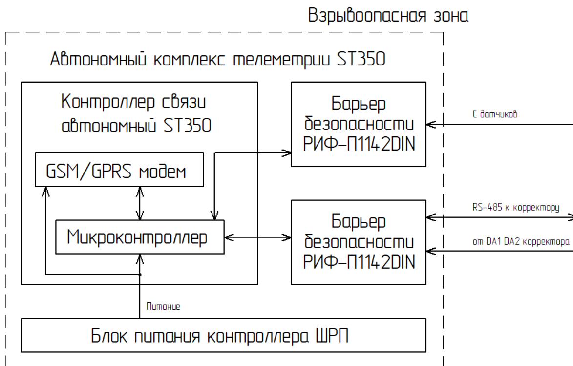
Рисунок 1.1 – Функциональная схема комплекса
