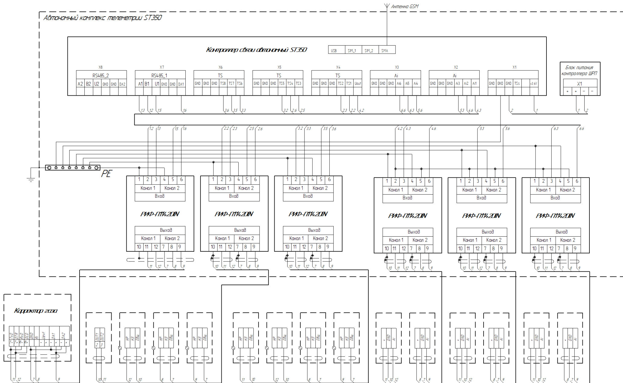
Рисунок Б.3 – Пример подключения комплекса продукт шифр 8-003 к одному электронному корректору (на примере ЕК270) и датчикам (8ТС и 6ТИ)
