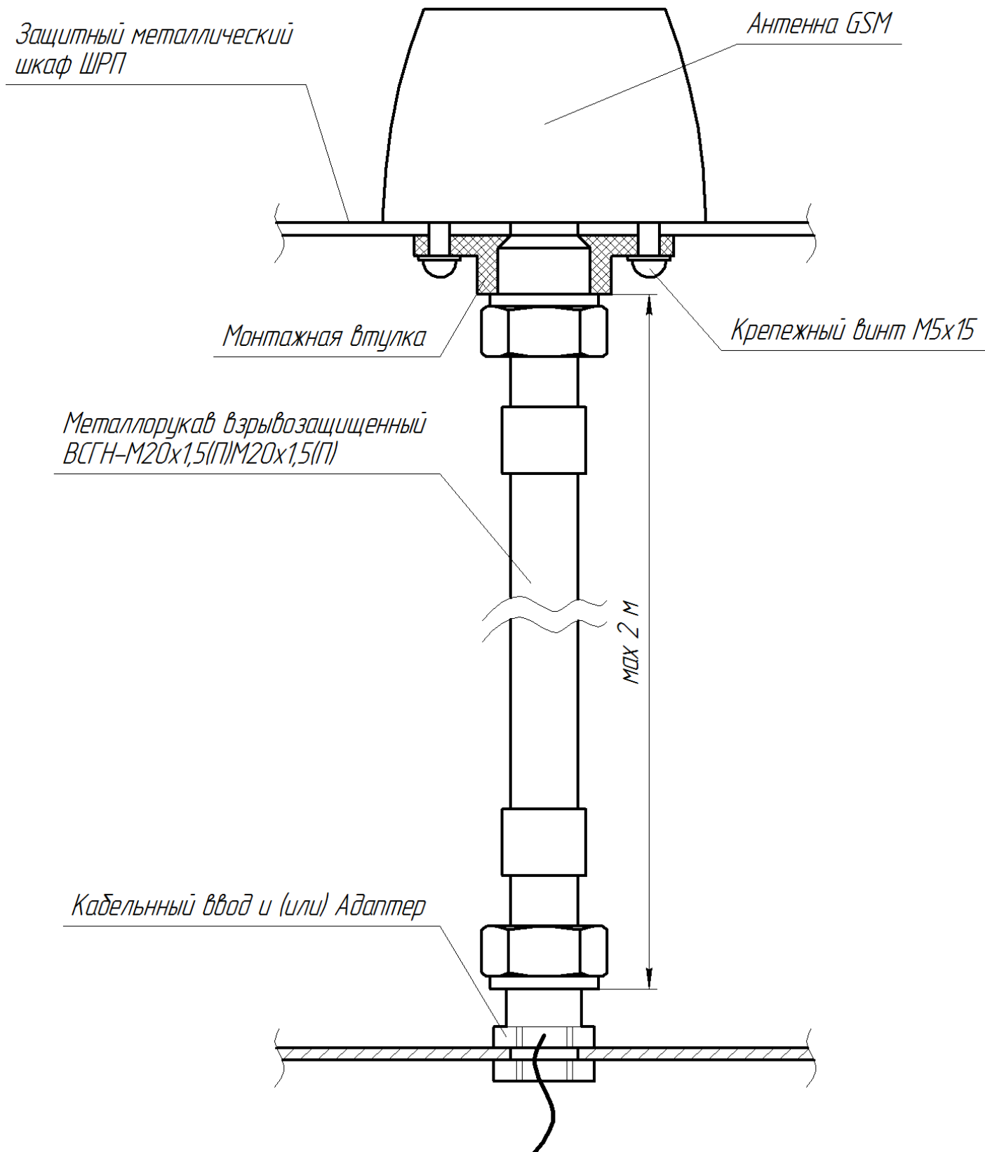
Рисунок В.1 – Схема установки выносной GSM-антенны
